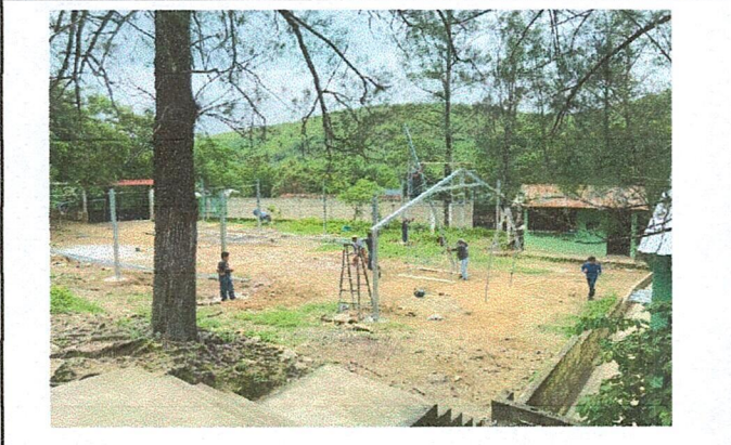
Foto 1: Trabajando en la estructura del área a techar.
